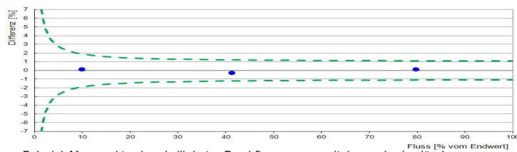
Beispiel: Messpunkte eines kalibrierten Durchflussmessers mit der maximal zulässigen Hüllkurve gemäß Definition
